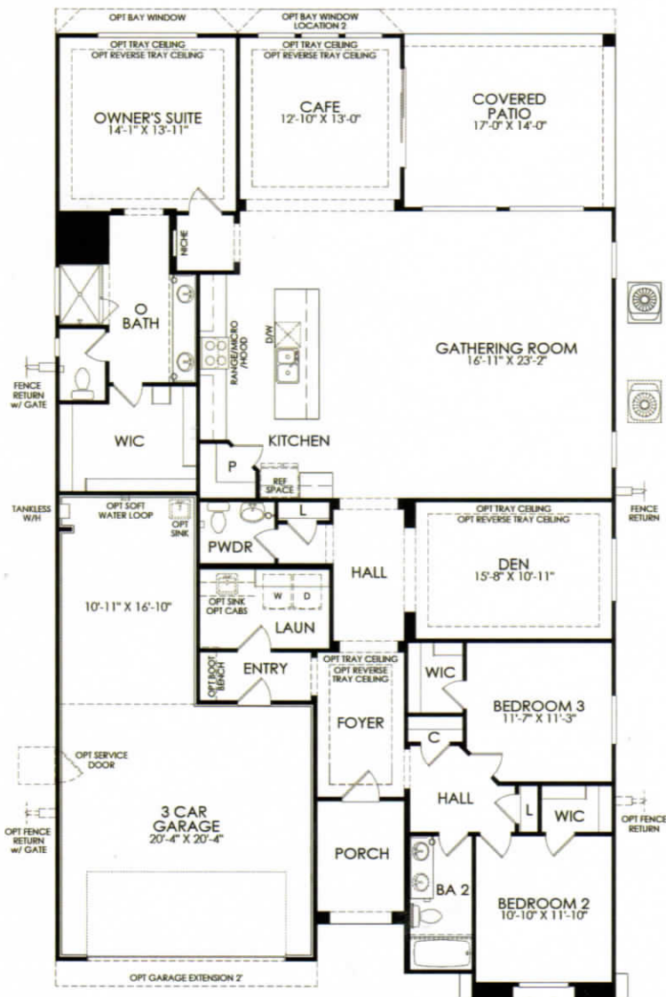
Elevation A
