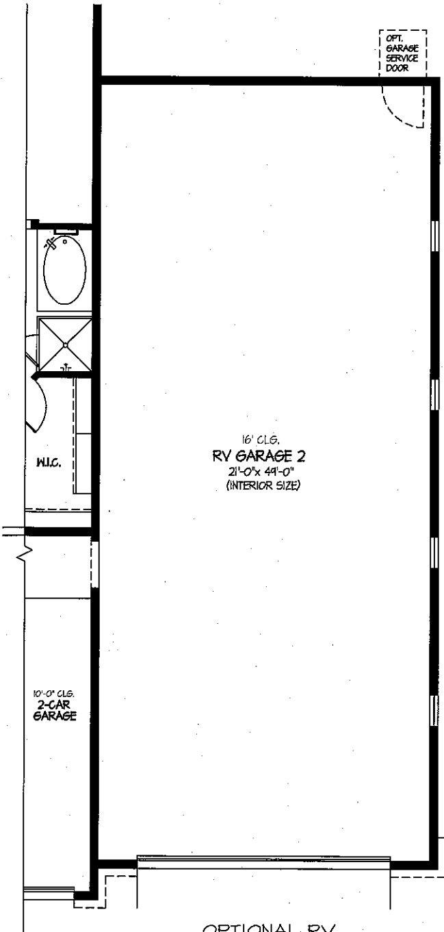
OPTIONAL RV GARAGE 2
