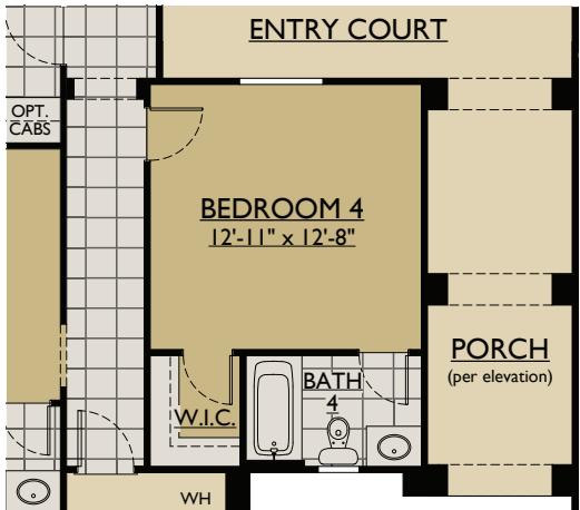
OPT. BEDROOM 4 & BATH 4 ILO SUITE
