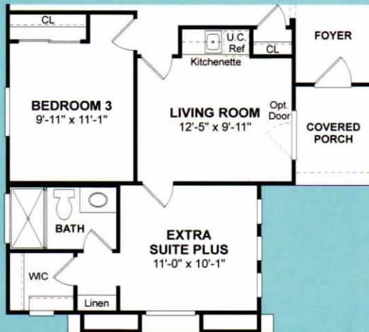
OPTIONAL EXTRA SUITE PLUS ILO BEDROOM 4
