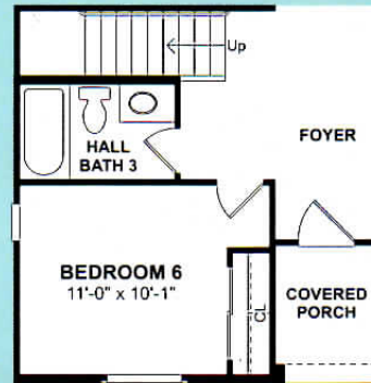
OPTIONAL BEDROOM 6/ HALL BATH 3
